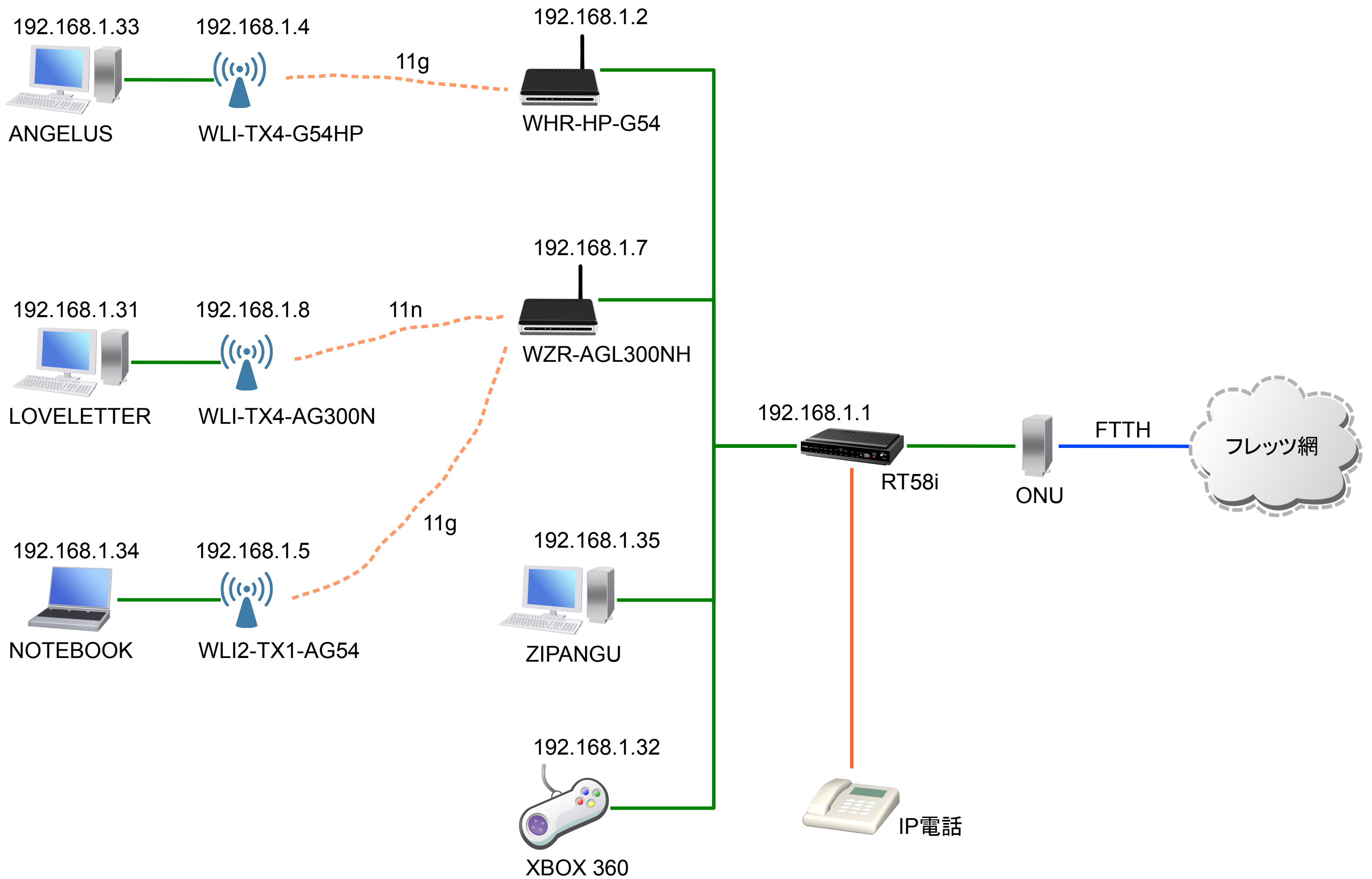
ネットワーク構成図 (2008-08-31)
