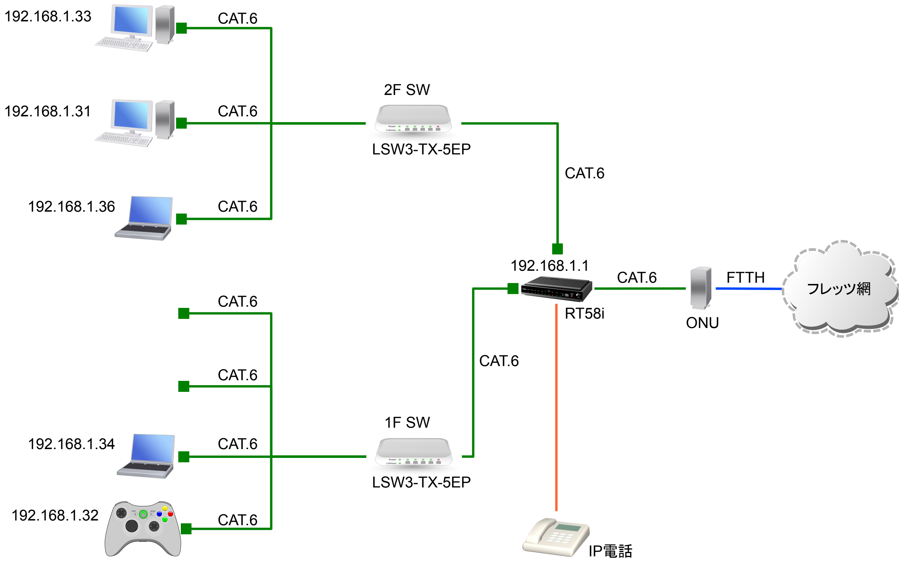
ネットワーク構成図 (2010-03-22)
