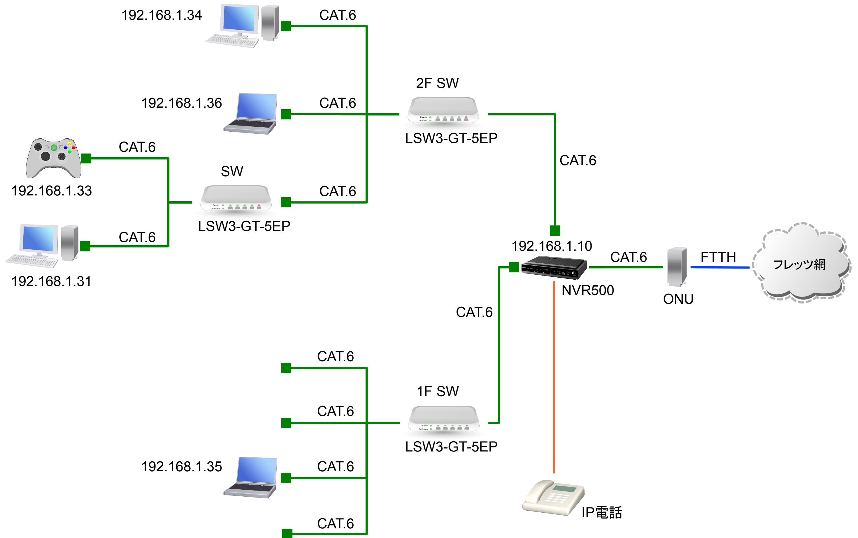
ネットワーク構成図 (2010-12-04)
