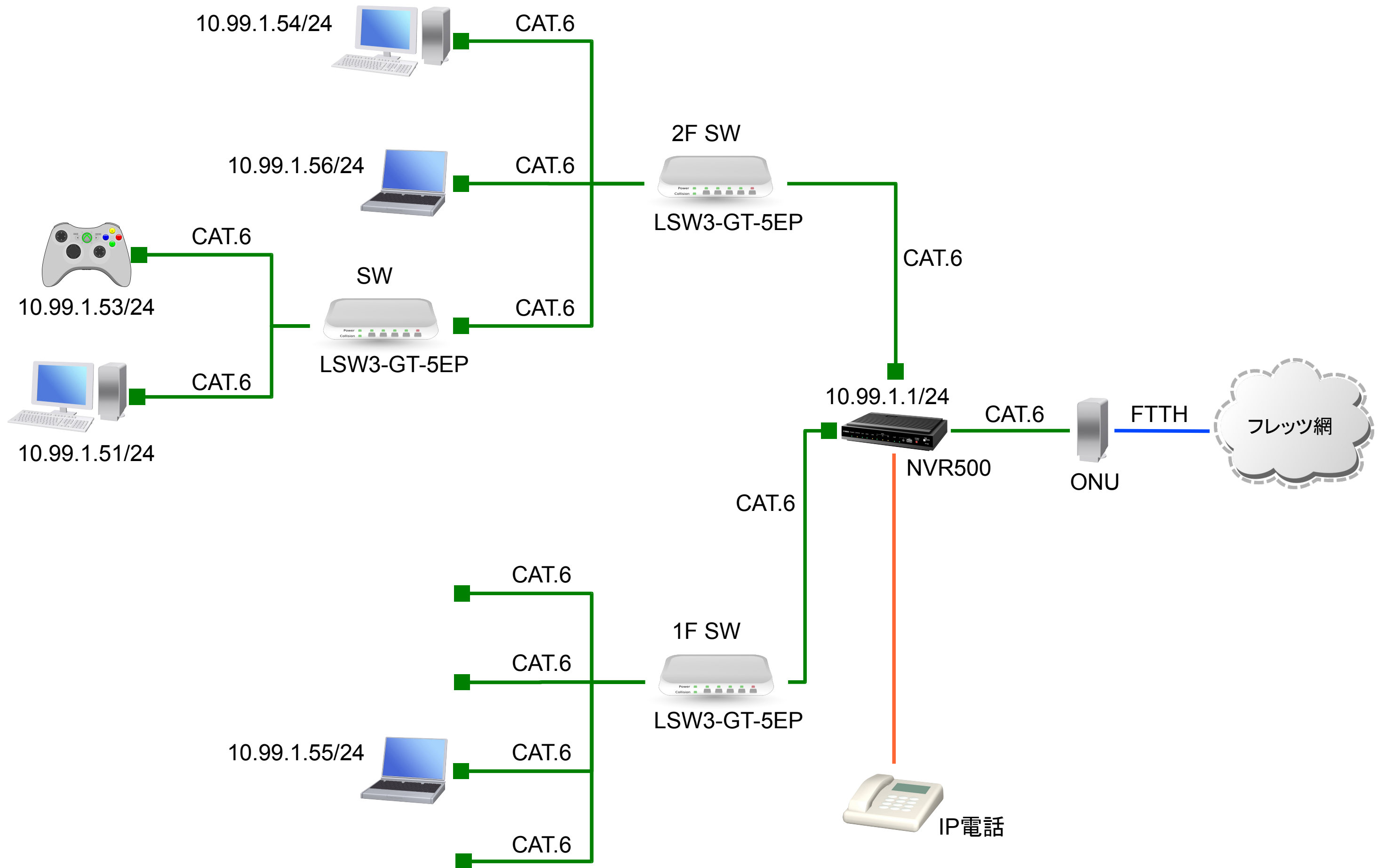
ネットワーク構成図 (2010-12-13)
