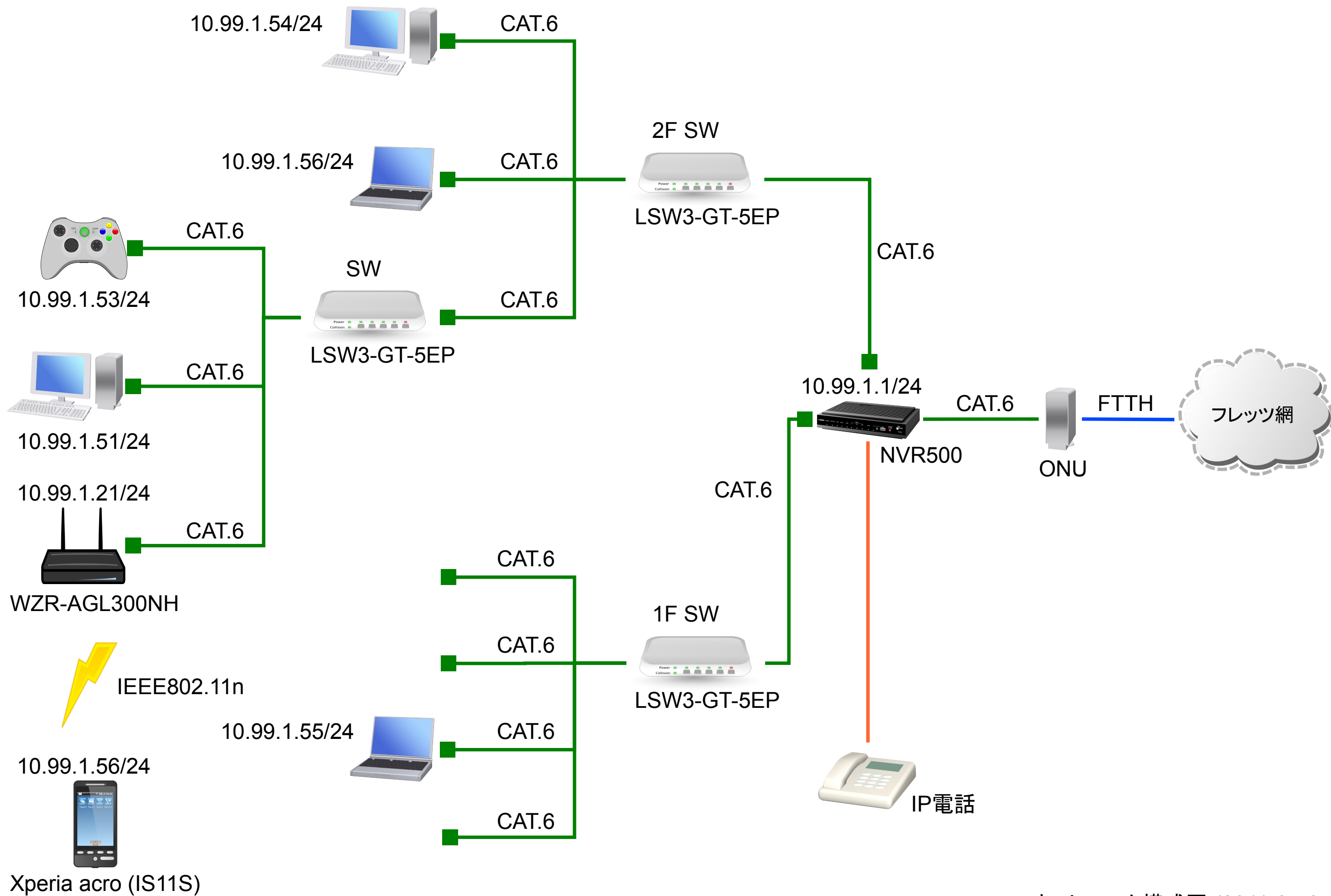
ネットワーク構成図 (2011-07-04)
