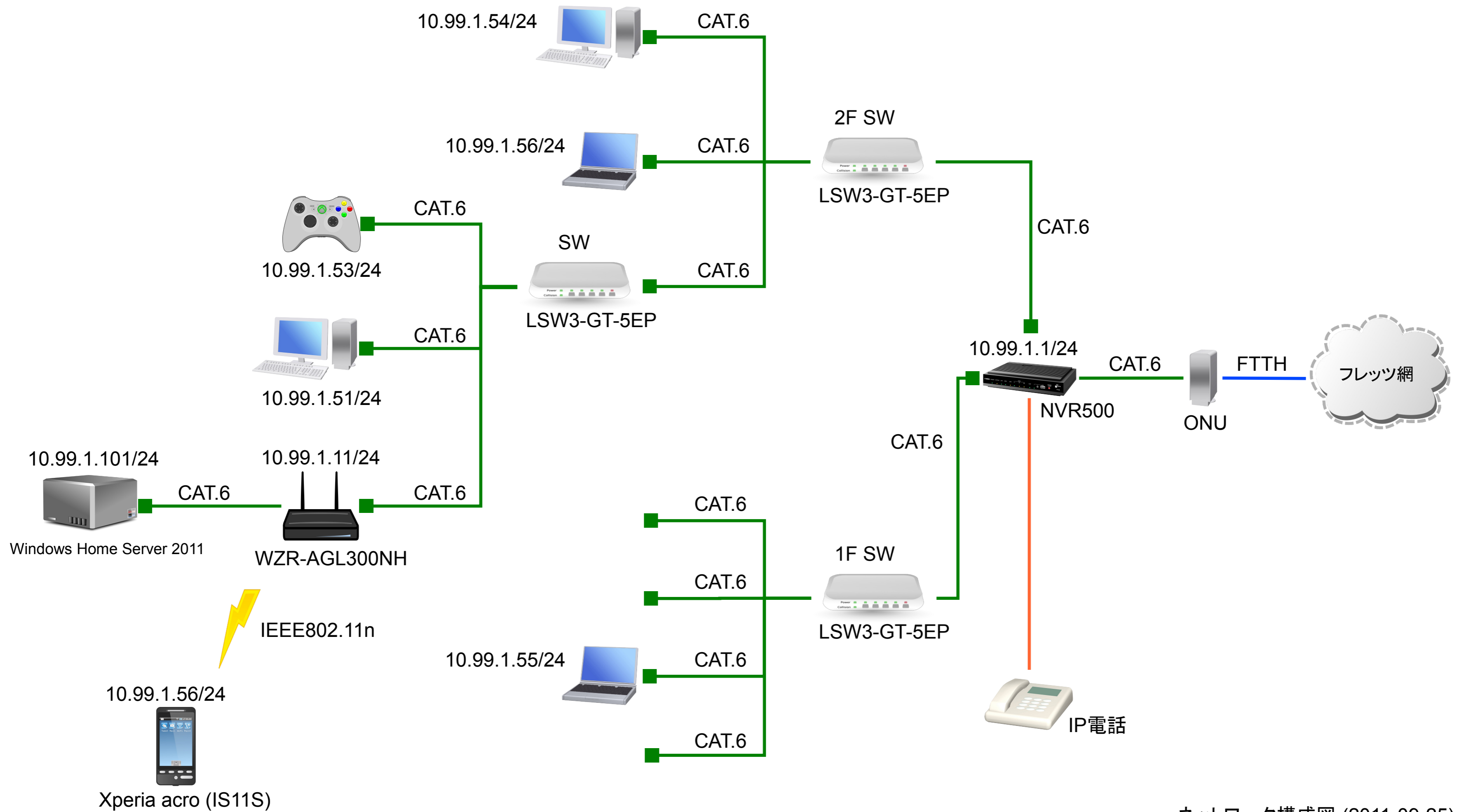
ネットワーク構成図 (2011-09-25)
