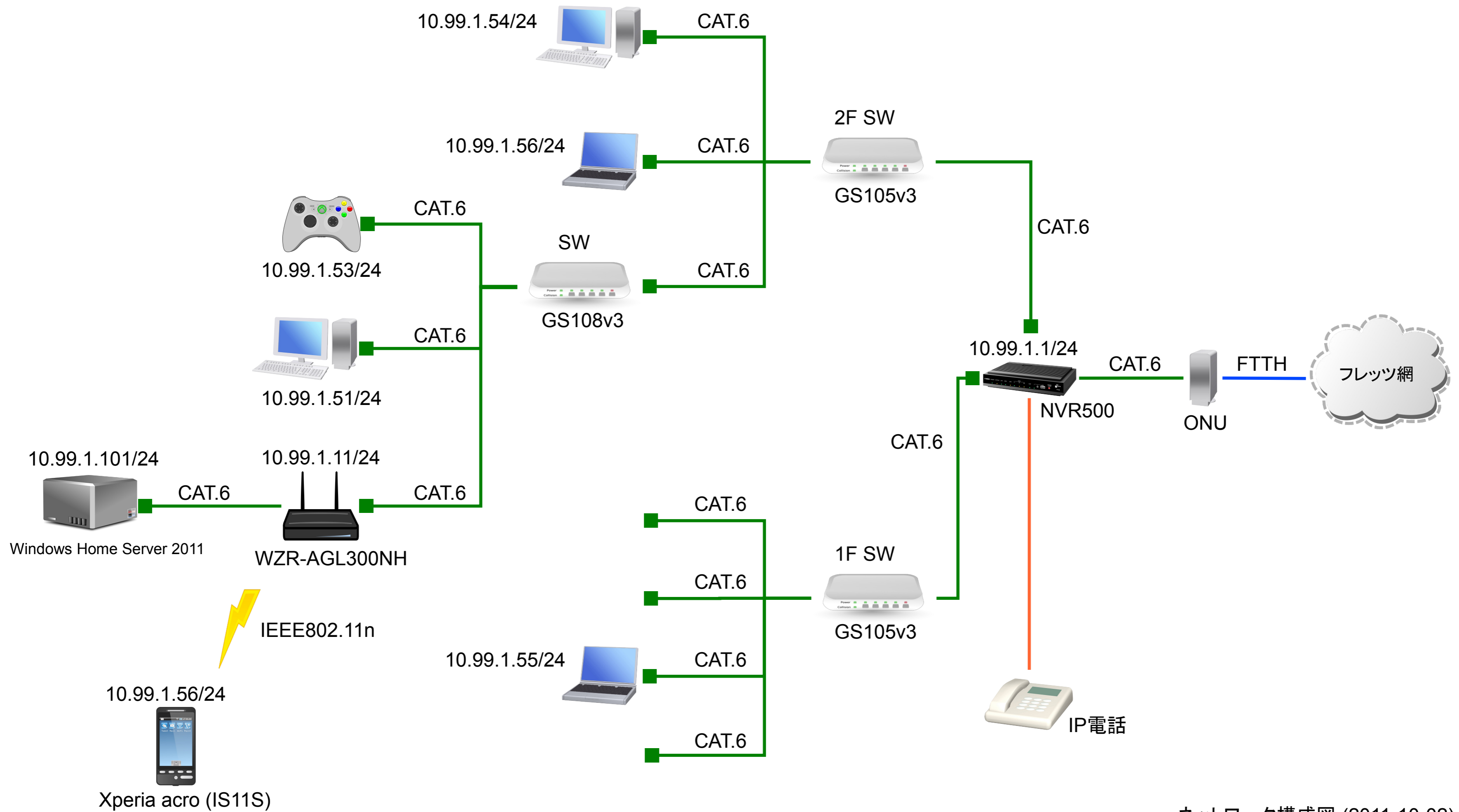
ネットワーク構成図 (2011-10-02)
