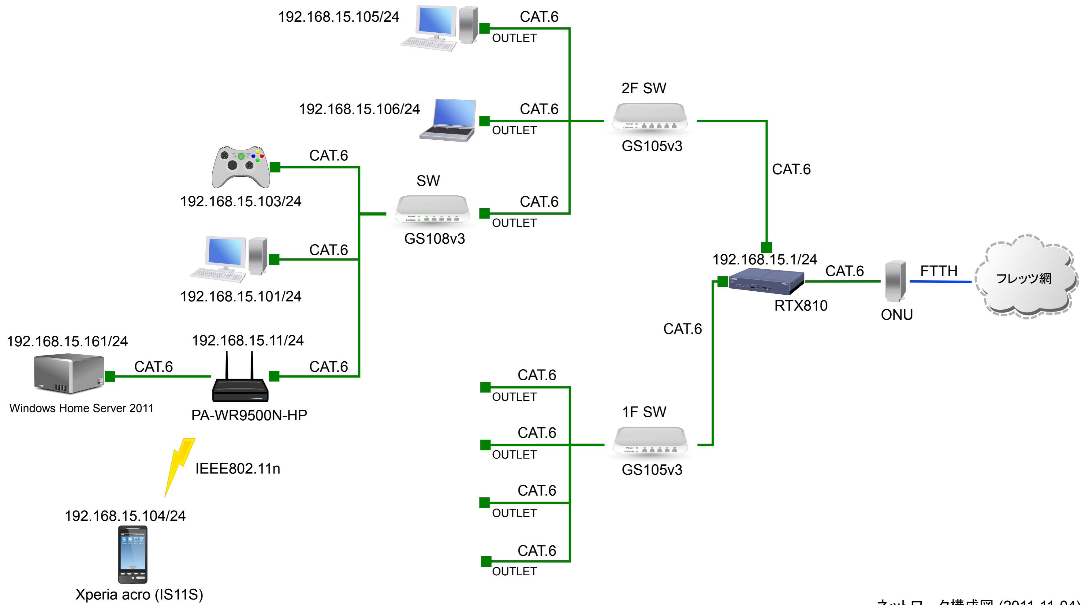
ネットワーク構成図 (2011-11-04)
