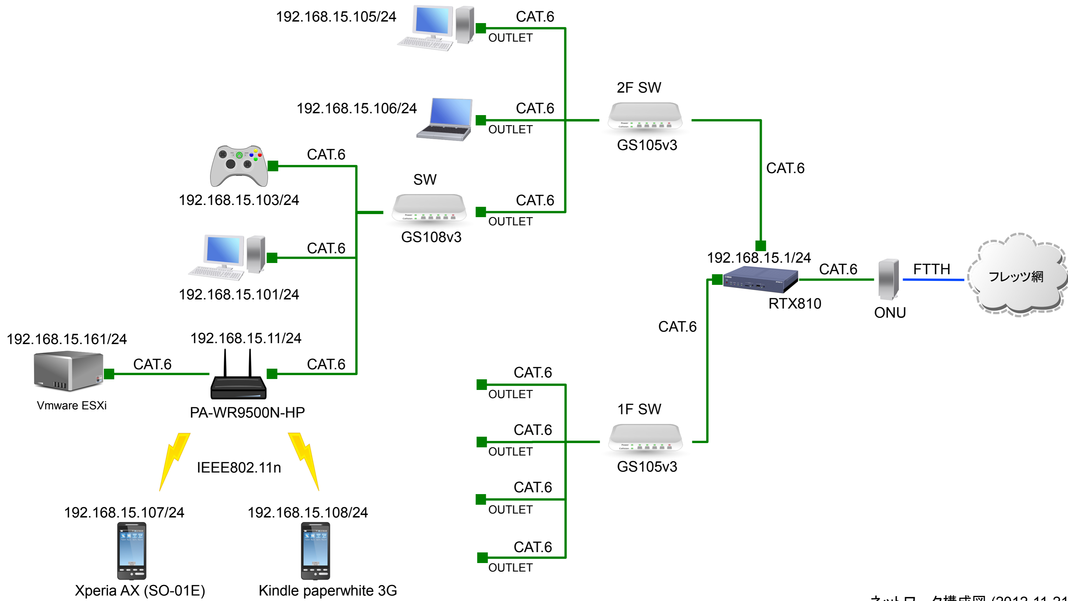
ネットワーク構成図 (2012-11-21)
